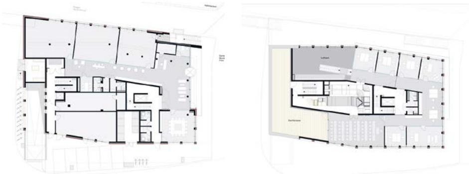
Die Grundrisse EG mit Zufahrt zur Tiefgarage (links) und 5. OG mit Dachterrasse (rechts).
