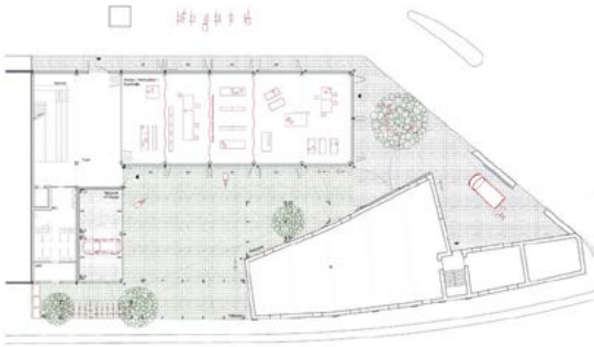
| Grundriss EG: Die Form des Bestandsgebäudes (rechts) wurde für den Neubau (links) gespiegelt und transformiert
