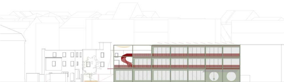
| Ansicht von der Speicherstraße: Fortführung des Straßenraums und Vermittlung der unterschiedlichen Nachbarbebauungen
